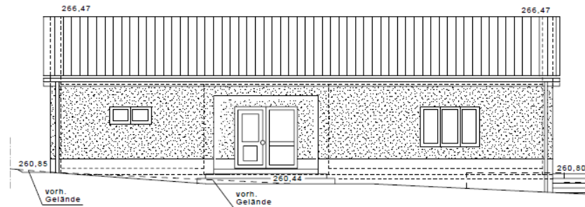
Ansicht Nord-West
